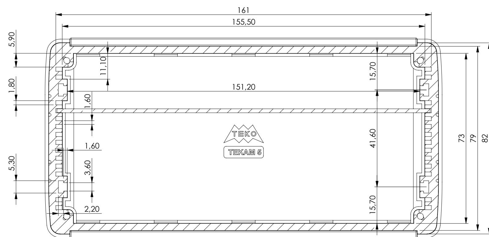
SEZIONE B-B
